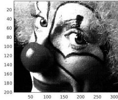
Figure 2.1: Image de clown 200 \times 320 pixels; la matrice correspondante est de rang 200.
