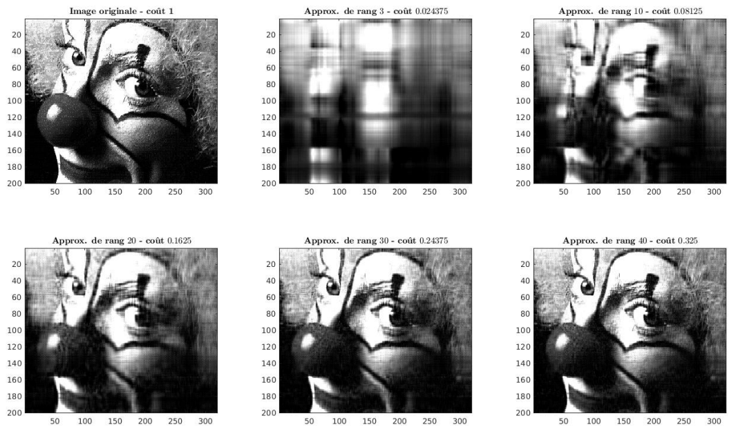
Figure 2.2: Image de clown 200 \times 320 et SVD tronquées avec k \in \{3, 10, 20, 30, 40\} ; le rang de chaque matrice est indiqué, ainsi que le ratio \frac{(m+n) \cdot k}{mn} .
